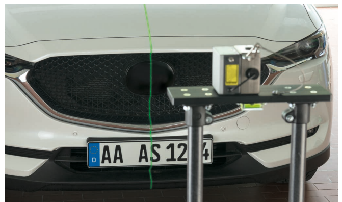
Laser a linea verde per allineamento con logo frontale e riferimenti centrali del veicolo
